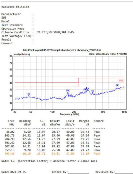
图 6-6 辐射测试水平方向
